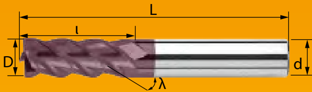
Фрезы четырехзубые
